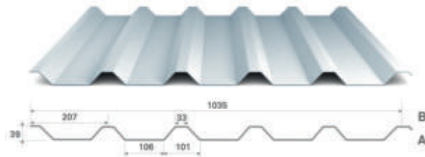
Trapezblech S35/207.PLUS
