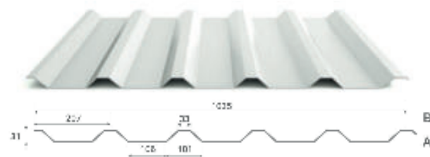
Trapezblech S35/207
