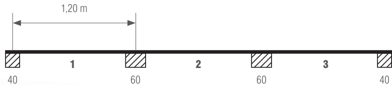
Belastungswerte nach Eurocode 3 (EN 1993-1-3): Profil in Negativlage, Dreifeldträger, Endauflagerbreite 40 mm, Zwischenaflagerbreite 60 mm
